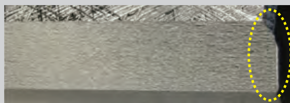
バリが発生
